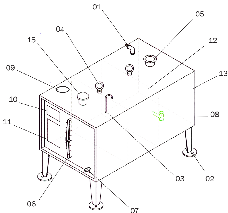
(油箱示意圖)
